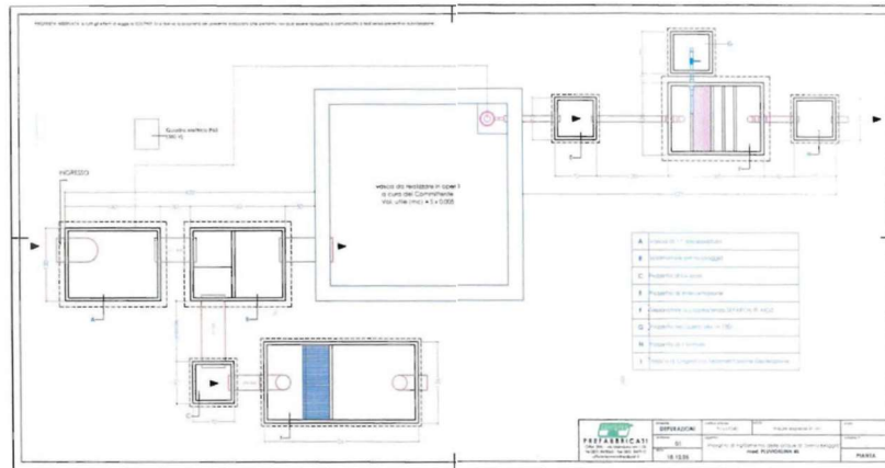
Schema in pianta riportato nella relazione e nella tavola 03
