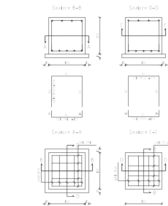
PLINTI 1-2-3-4-5-6-7-8-9-10 PLINTO TIPO SCALA 1:50
