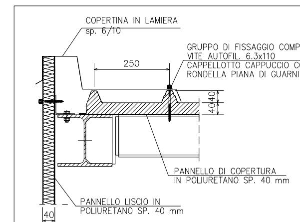
DETTAGLIO COLLEGAMENTO PANNELLI IN POLIURETANO SCALA 1:10
