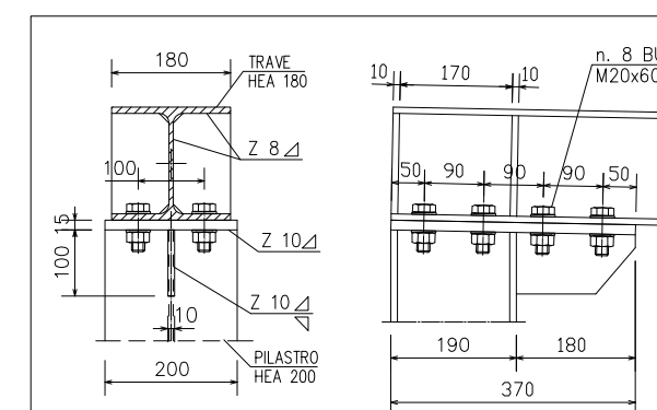
DETTAGLIO COLLEGAMENTO TRAVE -PILASTRO HEA200 SCALA 1:10
