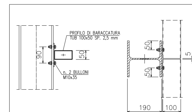
DETTAGLIO TYPICO FISSAGGIO PROFILO DI BARACCATURA SCALA 1:10
