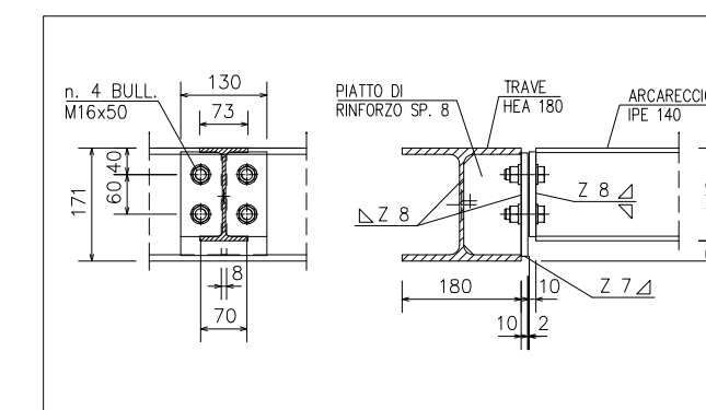
DETTAGLIO COLLEGAMENTO TRAVE -ARCARECCIO SCALA 1:10
