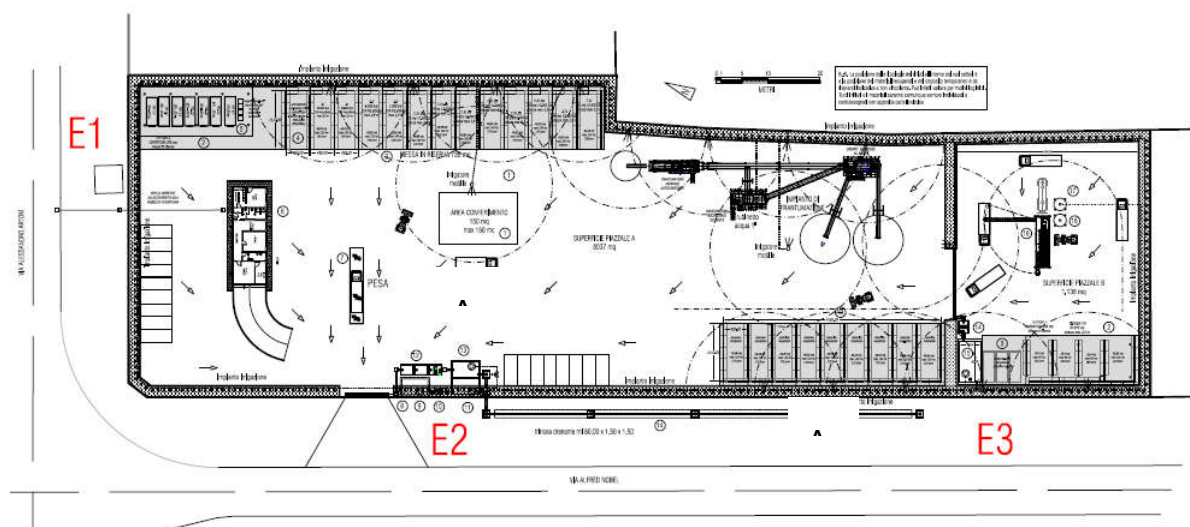
Figura 1 - planimetria con proposta punti di monitoraggio discontinuo dell'atmosfera
