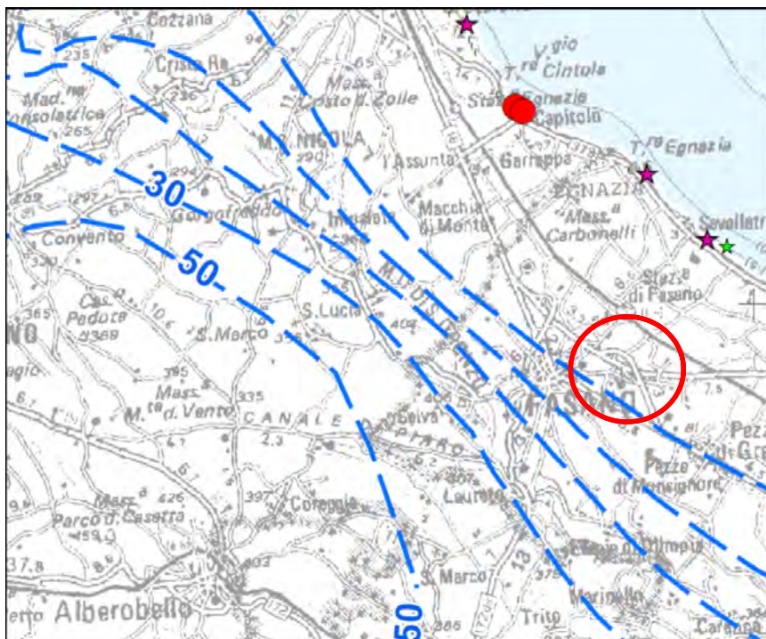
Fig. 4- Isopiezometrica dal PTA Puglia.
