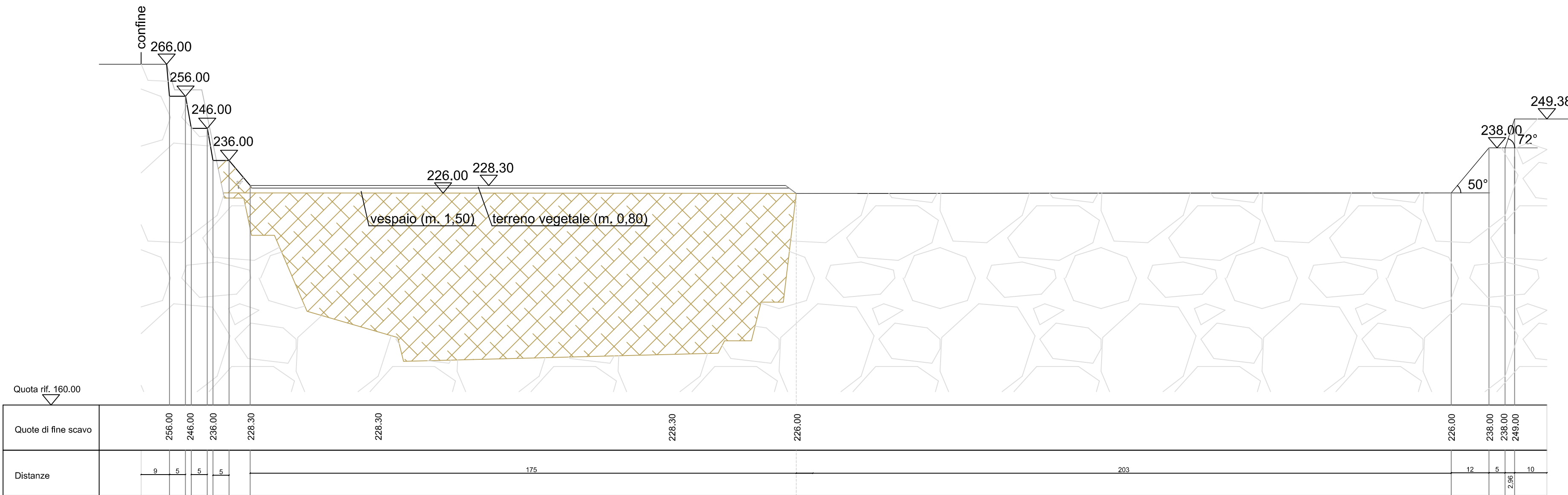
SEZIONE A-A' SCALA 1:1000
