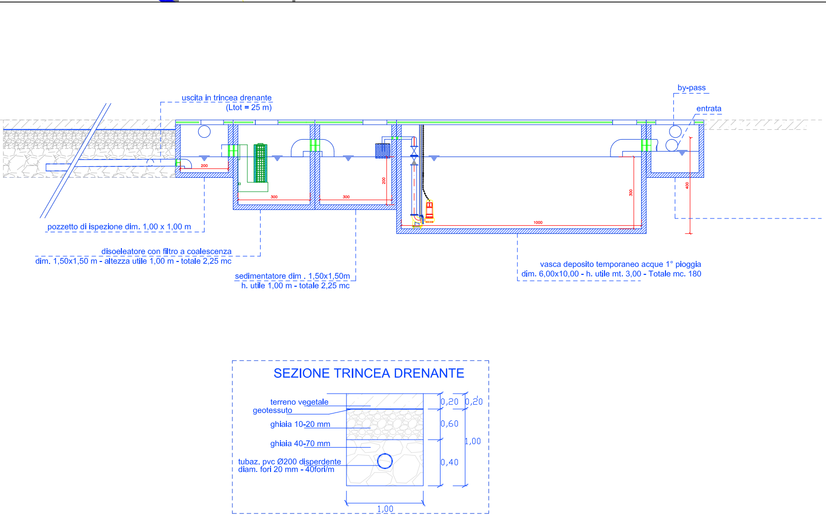
IMPIANTO TRATTAMENTO ACQUE PRIMA PIOGGIA E SUBIRRIGAZIONE
